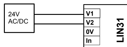
Podłączenie zasilania.
